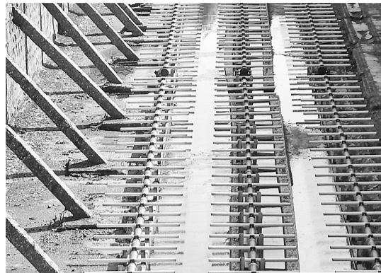
В одном из аэротенков уже установлены новые двойные аэрационные трубки
