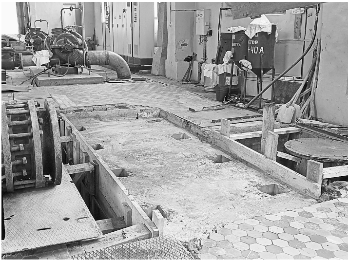
Фундамент под насосную установку готов
