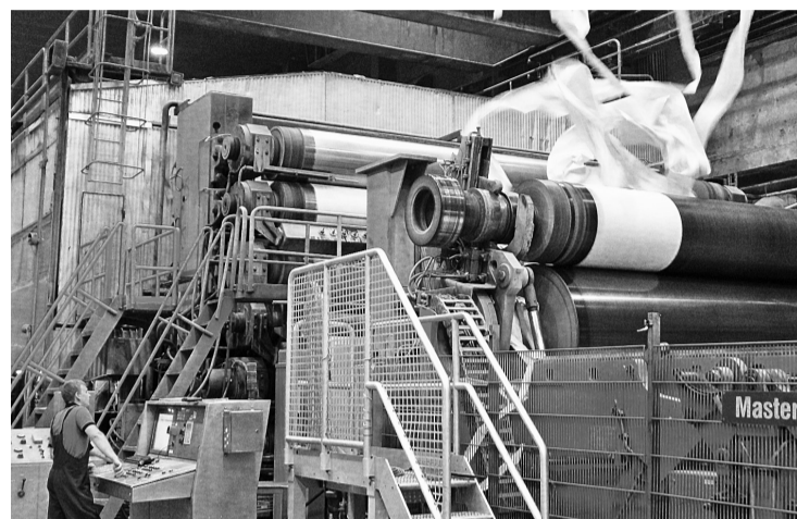
Сушильщик БДМ 6 разряда А.И. Мизёв производит заправку бумаги на тамбурный вал
