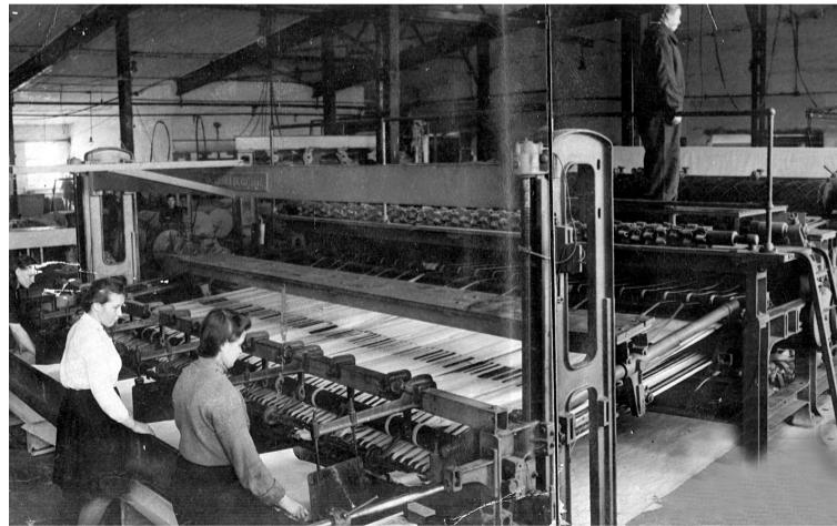
Ротационная саморезка для листовой газетной бумаги. Листохваты
