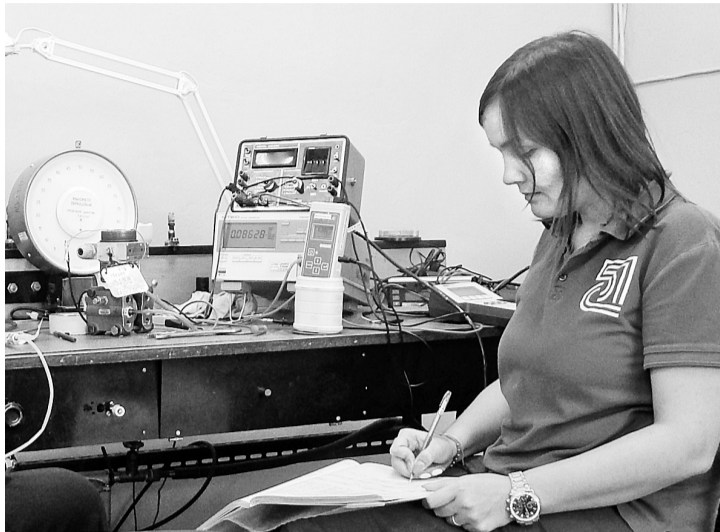
Калибровку проводит слесарь по КИПиА — А.В. Чейкаукас
