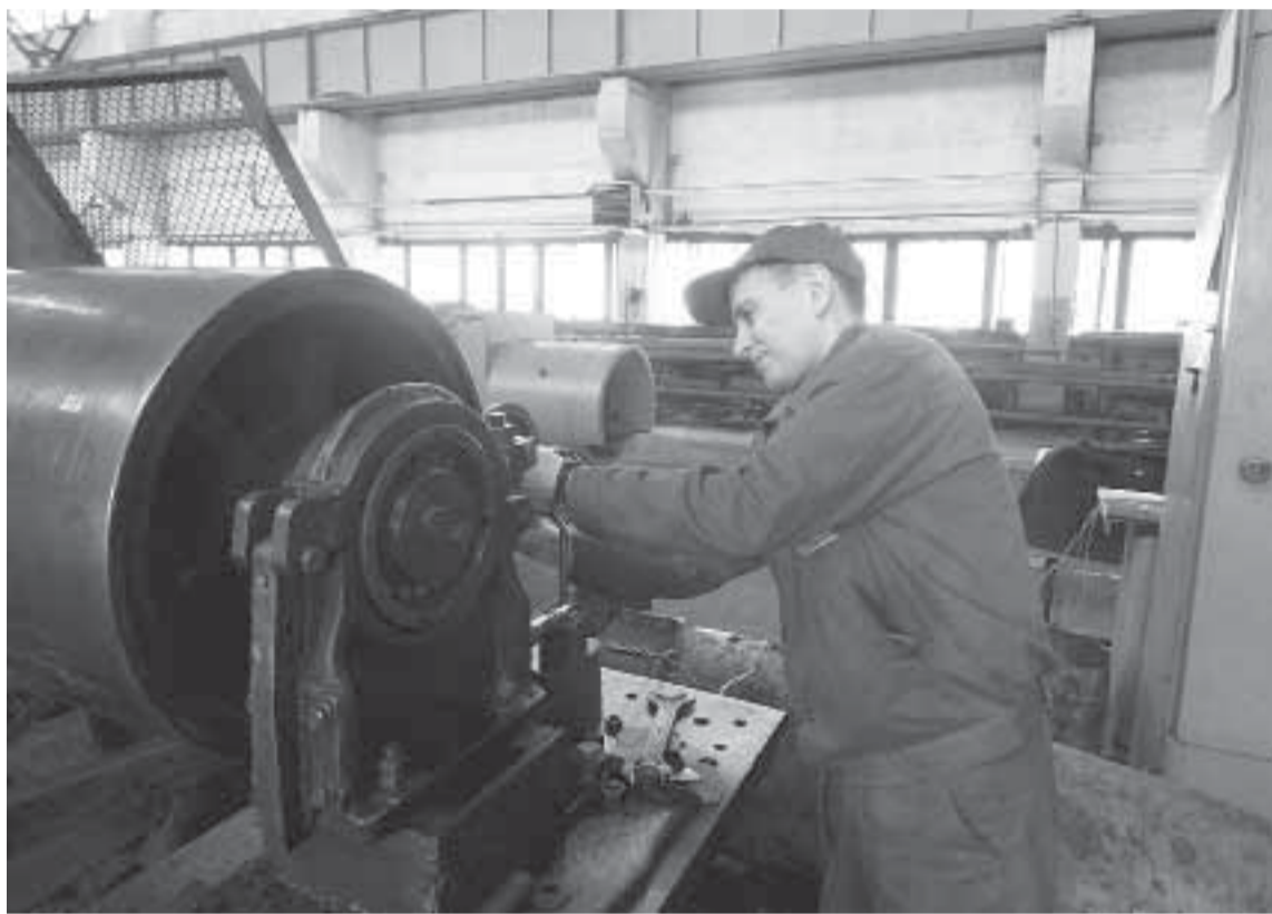
Лаборант ТДО 6 разряда А.М. Сандраков устанавливает датчики оборотов и датчики вибрации для проведения работы по балансировке вала.
